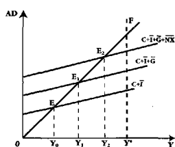
Рис.1 «Кейнсианский крест»
