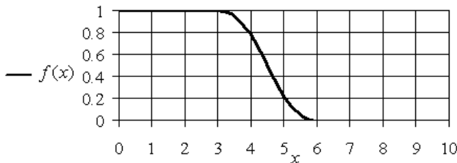
Рис. 1.11. График Z -образной функции принадлежности f_{z_2} для значений параметров A = 3, B = 6, P = 2
