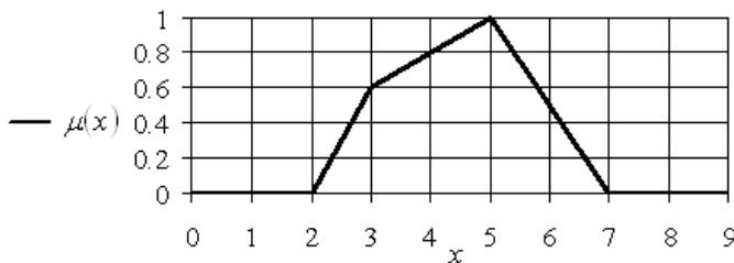
Рис. 1.6. График функции принадлежности выпуклого нечеткого множества
