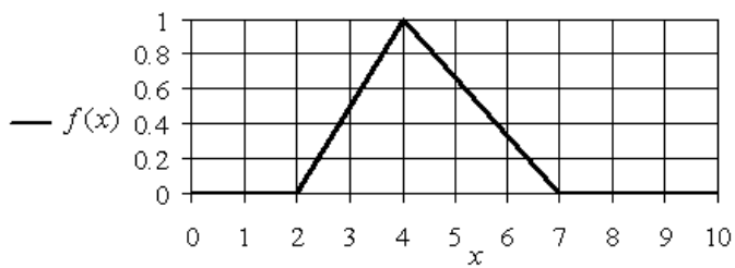
График функций принадлежности треугольной формы
