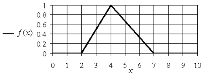
Рис. 1.8. График функций принадлежности треугольной формы Треугольная функция принадлежности в общем случае может быть аналитически задана следующим выражением:
