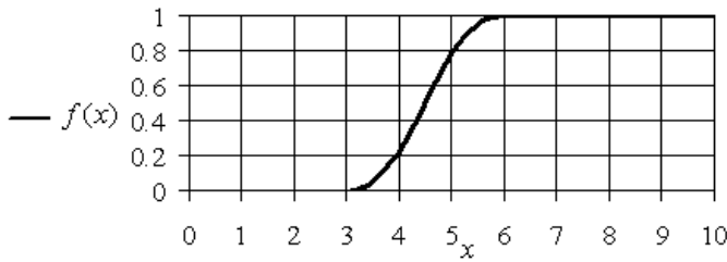
Рис. 1.13. График S-образной функций принадлежности f_{s_2} для значений параметров A = 3, B = 6, P = 2
