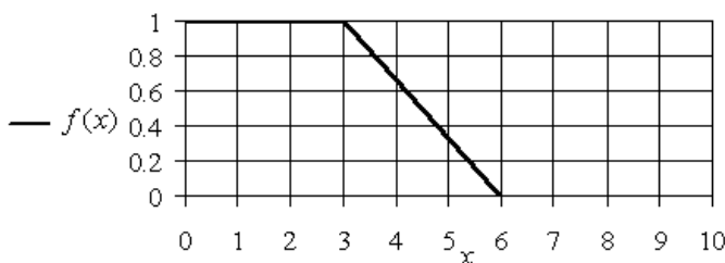
Рис. 1.16. График линейной Z -образной функции принадлежности для значений параметров A = 3, B = 6
