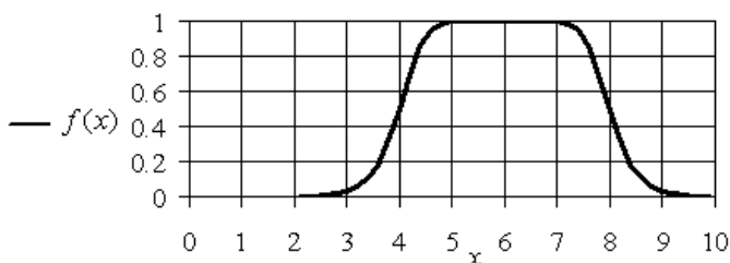
Рис. 1.20. График \Pi -образной функций принадлежности f_{\Pi_3} для значений параметров a = 2, b = 4, c = 6
