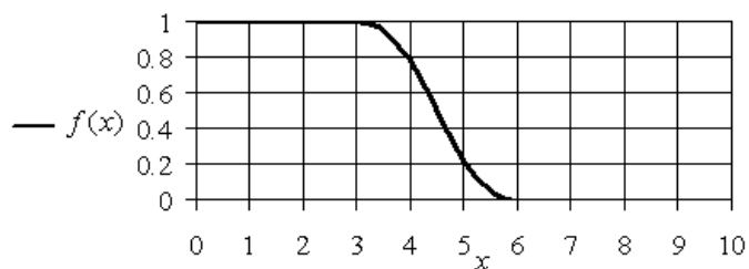
График Z-образной функции принадлежности f_x , для значений параметров A = 3, B = 6, P = 2
