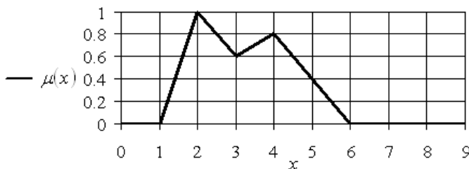
Рис. 1.7. График функции принадлежности невыпуклого нечеткого множества
