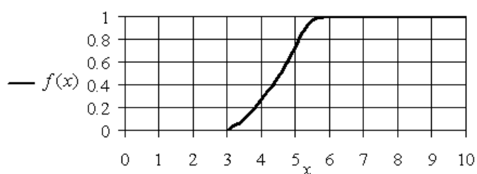
График S-образной функции принадлежности f_a для значений параметров A = 3, B = 6
