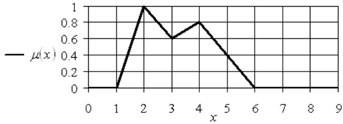
График функции принадлежности невыпуклого нечеткого множества
