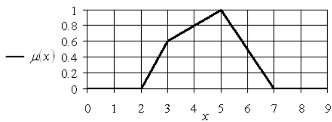
График функции принадлежности выпуклого нечеткого множества
