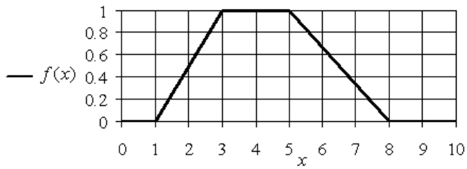
График функций принадлежности трапецевидной формы
