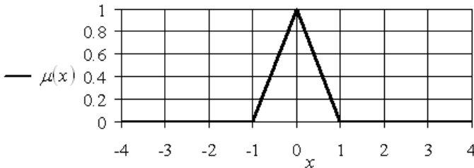
Рис. 1.3. Графическое изображение функции принадлежности бесконечного нечеткого множества «действительное число, приближенно равное нулю»
