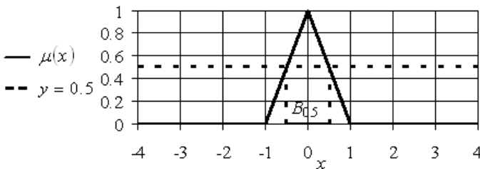
Рис. 1.4. Графическое изображение функции принадлежности бесконечного нечеткого множества 0.5-уровня «действительное число, приближенно равное нулю»
