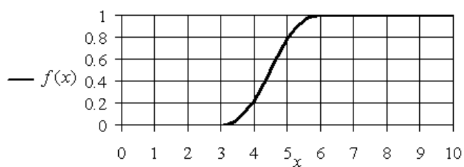
График S-образной функций принадлежности f_{s_1} для значений параметров A = 3, B = 6, P = 2
