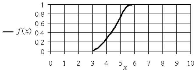
Рис. 1.12. График S-образной функции принадлежности f_a для значений параметров A = 3, B = 6
