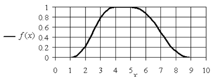
График П-образной функции принадлежности f_{\Pi_1} для значений параметров a = 1 , b = 4 , c = 5 , d = 9
