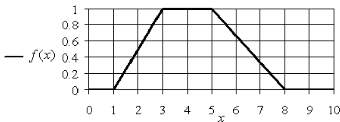
Рис. 1.9. График функций принадлежности трапециевидной формы
