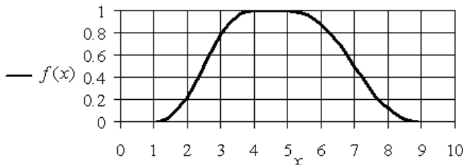
Рис. 1.18. График \Pi -образной функции принадлежности f_{\Pi_1} для значений параметров a = 1, b = 4, c = 5, d = 9
