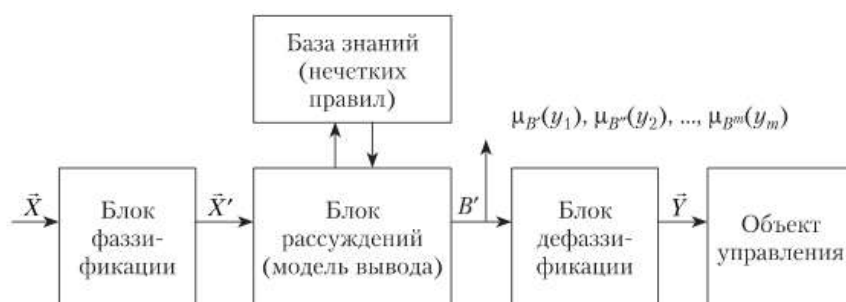
Архитектура нечеткой экспертной системы
