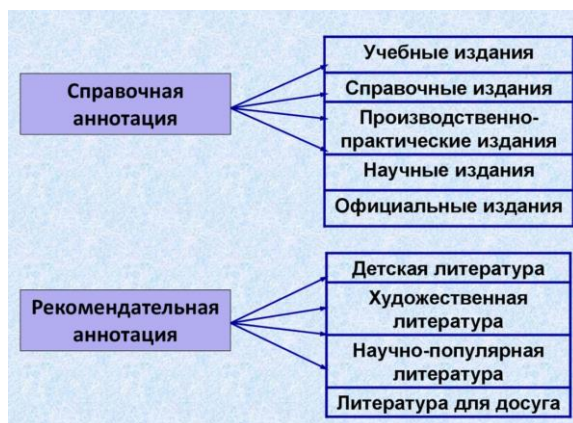
рис.3 Виды аннотаций
