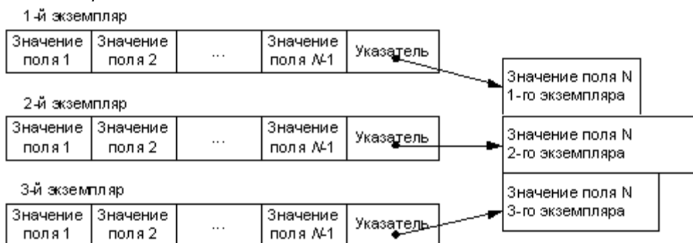
Рис. 9.2. Представление полей переменной длины
