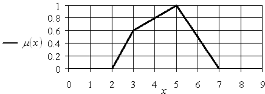
Рис. 1.6. График функции принадлежности выпуклого нечеткого множества
