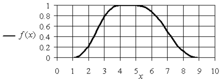
График \Pi -образной функции принадлежности f_{\Pi_1} для значений параметров a = 1 , b = 4 , c = 5 , d = 9
