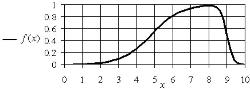
Рис. 1.19. График \Pi -образной функции принадлежности f_{\Pi_3} для значений параметров b_1 = 0.62, c_1 = -3, b_2 = -3, c_2 = 27
