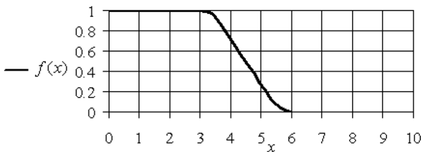
Рис. 1.10. График Z -образной функции принадлежности f_{z_1} Для значений параметров A = 3, B = 6
