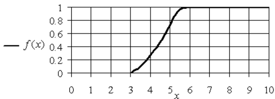
График S-образной функции принадлежности f_{s_1} для значений параметров A = 3, B = 6
