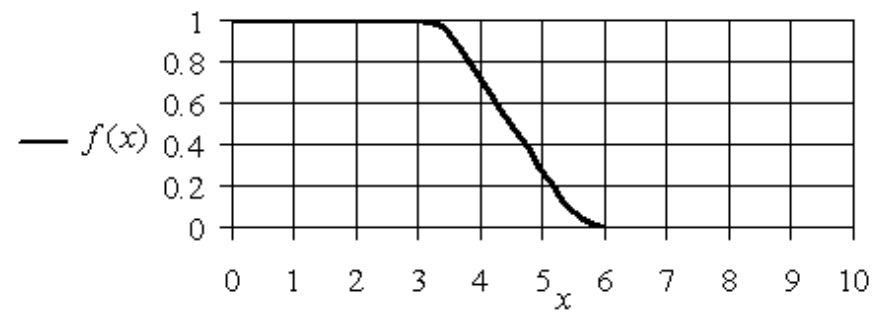
График Z -образной функции принадлежности f_{z_1} Для значений параметров A = 3, B = 6
