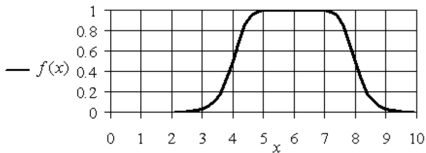
График \Pi -образной функций принадлежности f_{\Pi_3} для значений параметров a = 2, b = 4, c = 6
