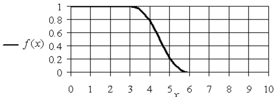
Рис. 1.11. График Z -образной функции принадлежности f_{z_1} для значений параметров A = 3, B = 6, P = 2
