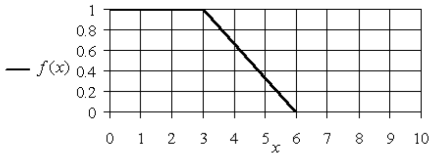
График линейной Z-образной функции принадлежности для значений параметров A = 3 , B = 6
