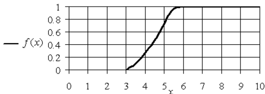
Рис. 1.12. График S-образной функции принадлежности f_a для значений параметров A = 3, B = 6
