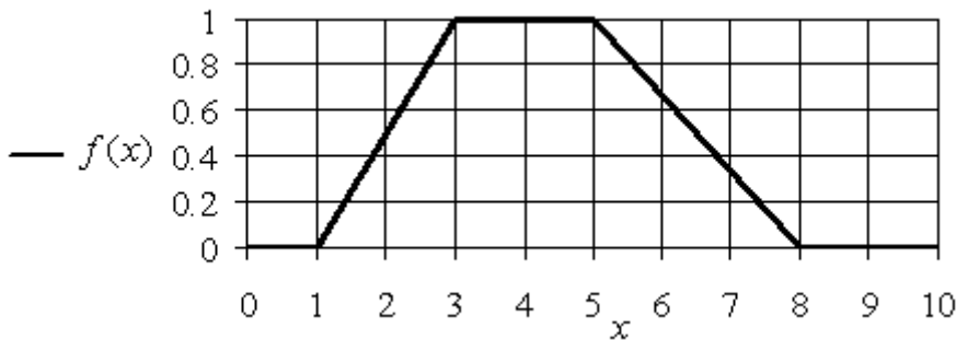
Рис. 1.9. График функций принадлежности трапециевидной формы
