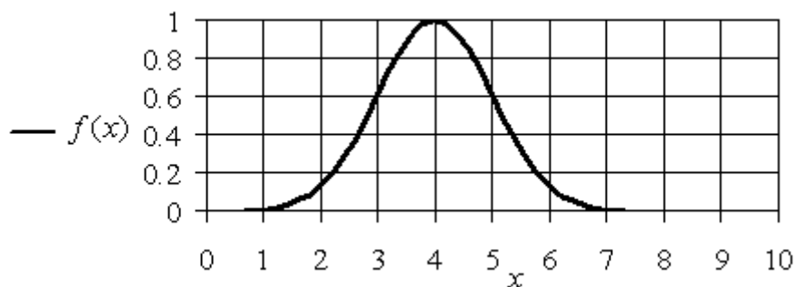
График \Pi -образной функции принадлежности f_{\Pi_4} для значений параметров \sigma = 1, c = 4
