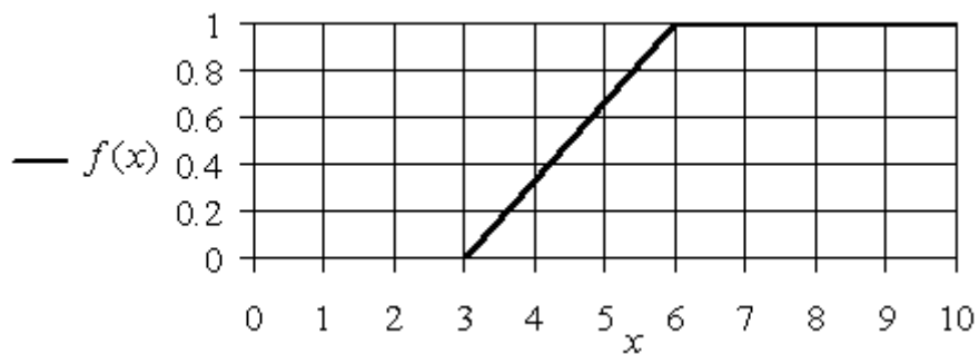
График линейной S-образной функции принадлежности для значений параметров a = 3 , b = 6
