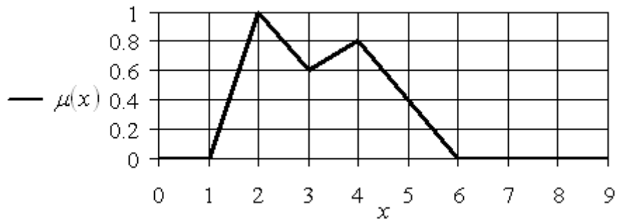
График функции принадлежности невыпуклого нечеткого множества
