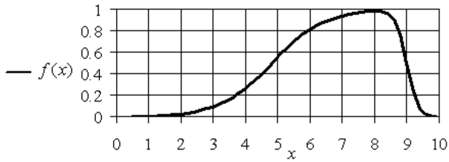
График \Pi -образной функции принадлежности f_{\Pi_3} для значений параметров b_1 = 0.62, c_1 = -3, b_2 = -3, c_2 = 27
