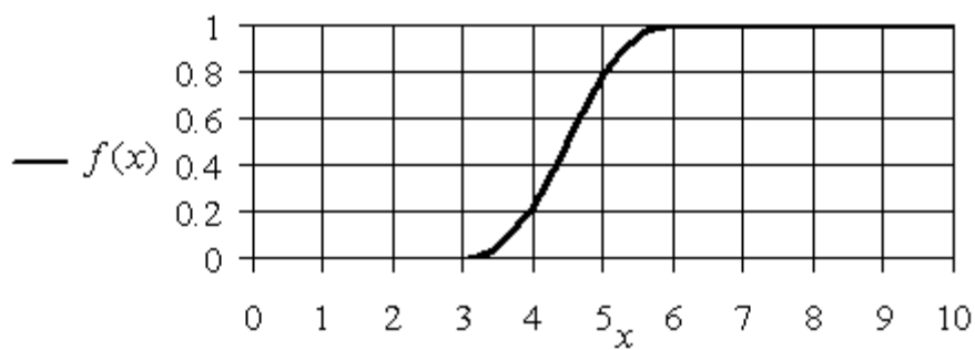
График S-образной функций принадлежности f_{s_2} для значений параметров A = 3, B = 6, P = 2
