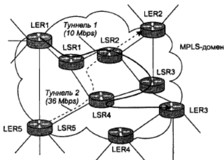
Рисунок. Два типа TE-туннелей в технологии MPLS.
