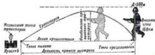
Рис. 3. Прямой выстрел
