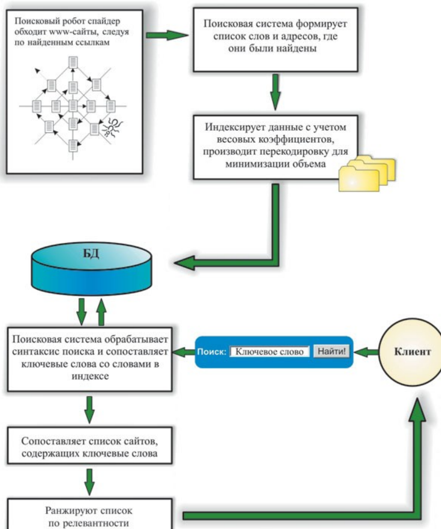
Рис. Роботы-пауки просматривают информационное наполнение Web-страниц и создают индексируемую базу поиска по ключевым словам, а затем по запросу пользователя выдают ранжированный по релевантности список сайтов.
