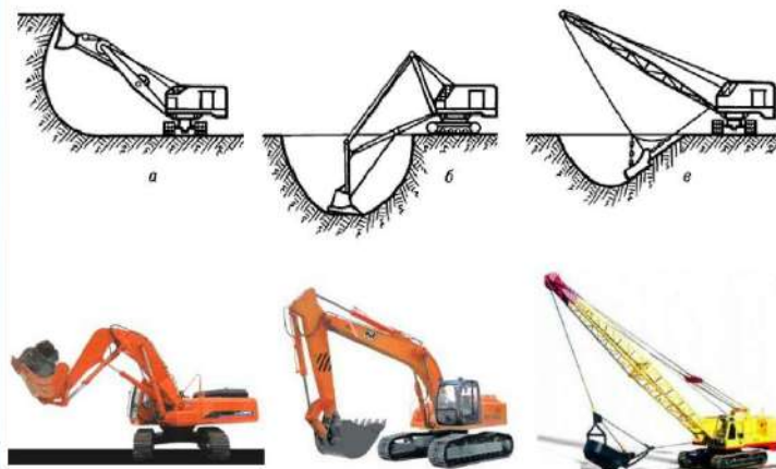
а – прямая лопата; б – обратная лопата; в - драглайн
