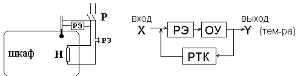
Рис. 1.3 Пример 3. Схема АСР температуры с измерительным мостом.
