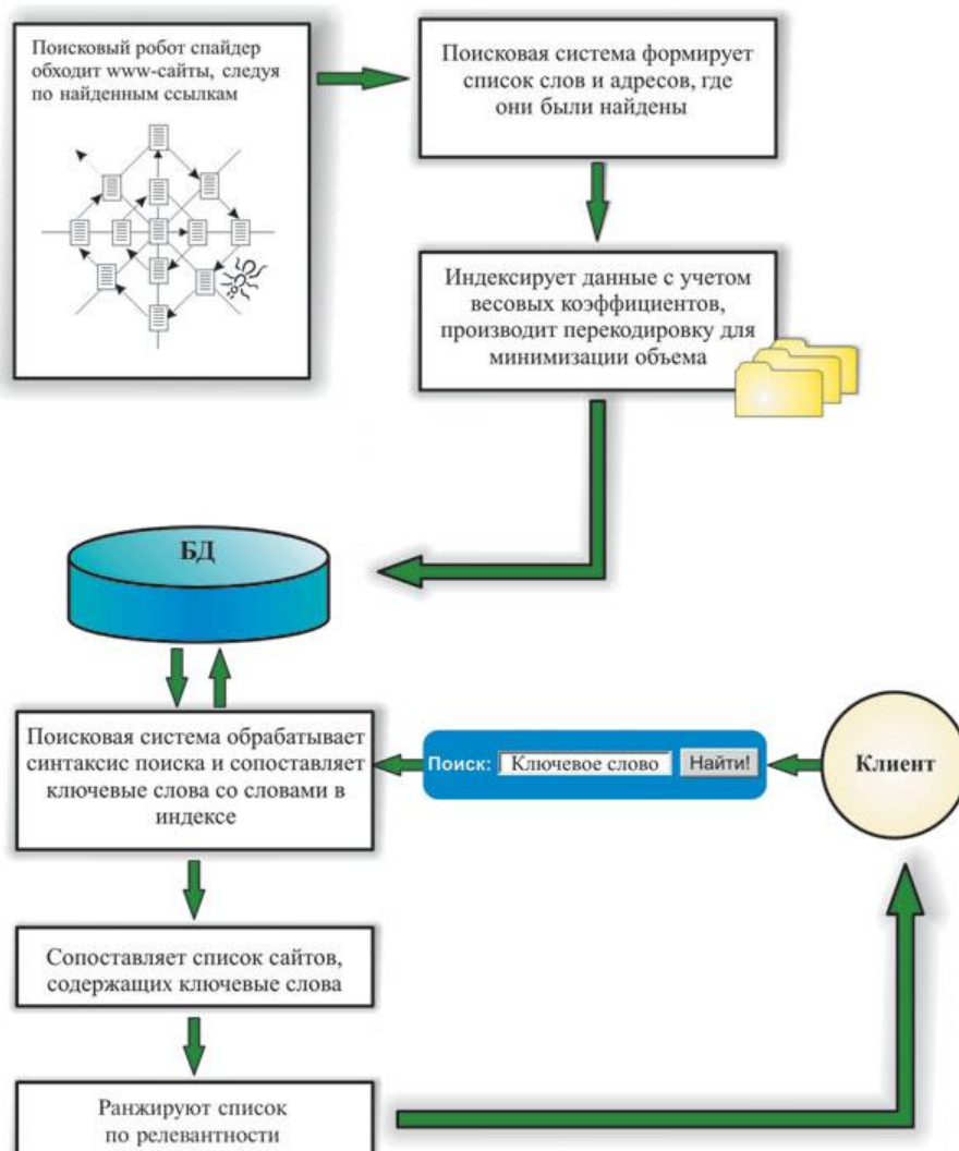
Рис.Роботы-пауки просматривают информационное наполнение Web-страниц и создают индексированную базу поиска по ключевым словам, а затем по запросу пользователя выдают ранжированный по релевантности список сайтов.
