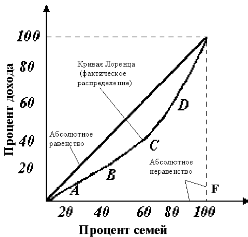
Рис 8. Джини-коэффициент
