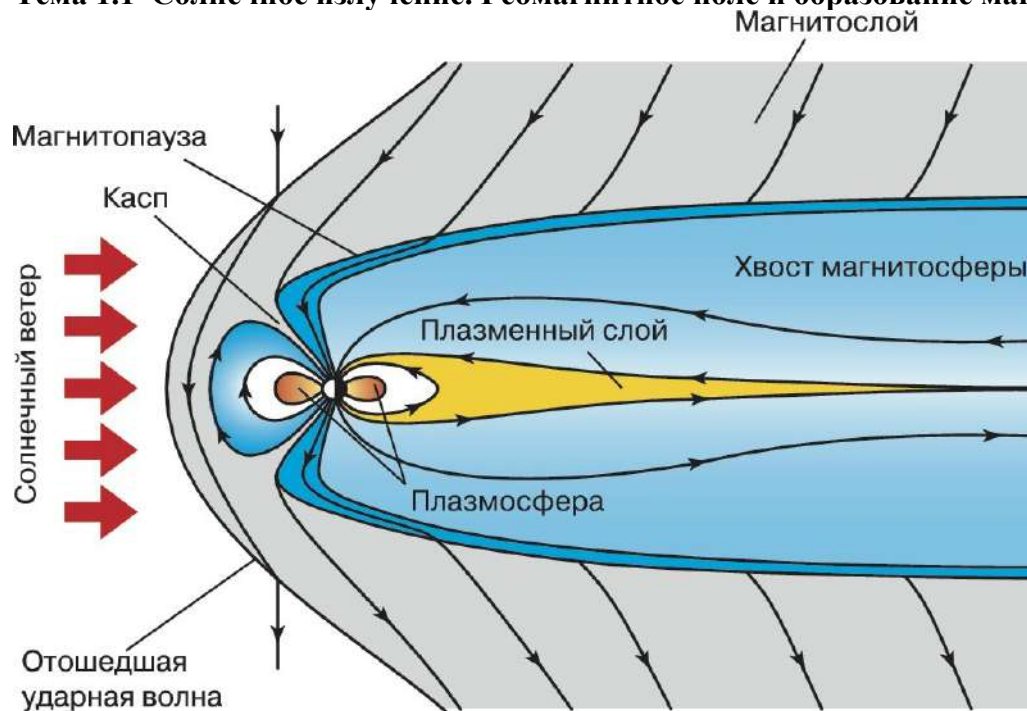
Рисунок 1. Магнитное поле Земли.
