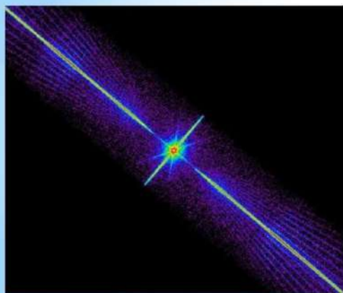
Рисунок 4. Рентгеновское излучение.
