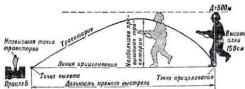
Рис. 3. Прямой выстрел
