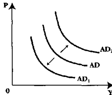
Рис. Неченовые факторы сдвига кривой AD
