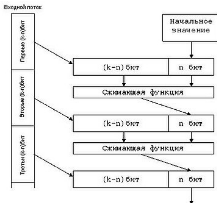
Рис 1. Итеративная последовательная схема
