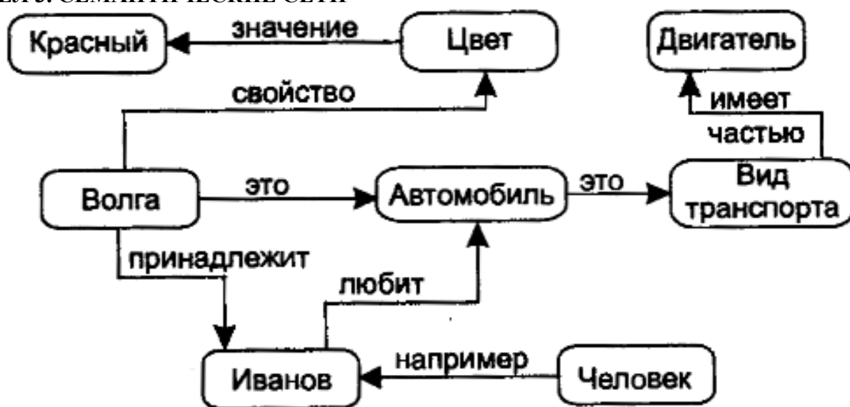
Рис. 1.1. Семантическая сеть
