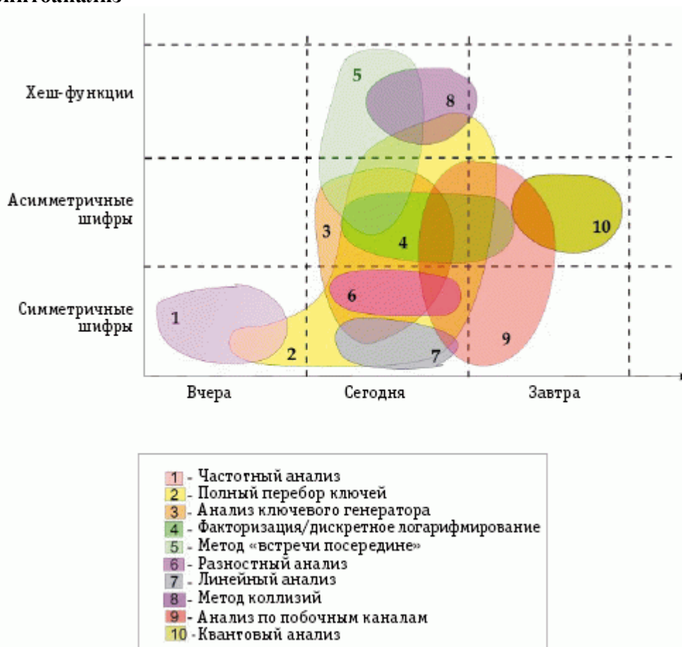
Рис. 1. Методы криптоанализа
