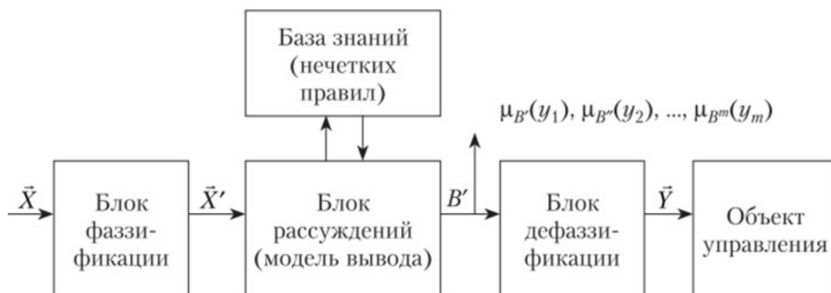
Архитектура нечеткой экспертной системы
