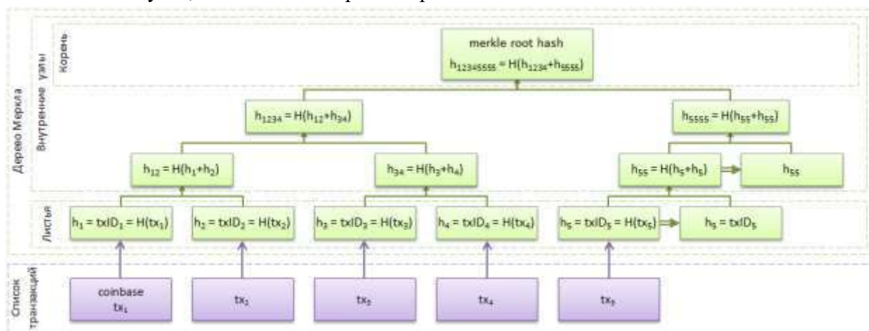
Рис.8. Пример схемы определения корня дерева Меркла ( H(M) = \text{SHA256}(\text{SHA256}(M)) )
