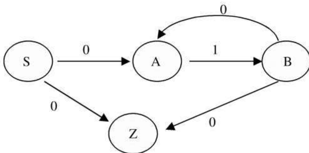
Конечный автомат
