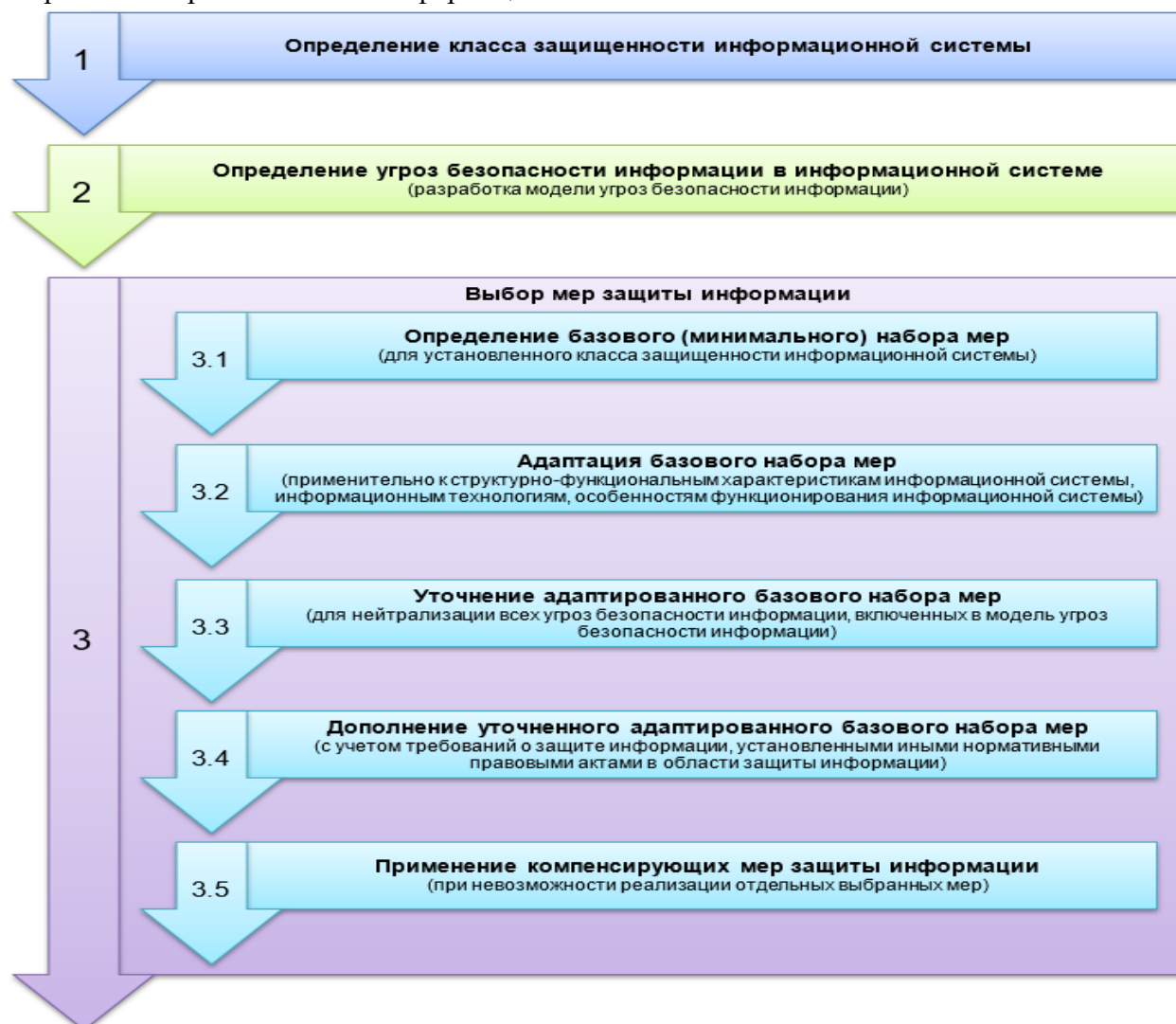
Рис.4. Порядок выработки мер обеспечения информационной безопасности
