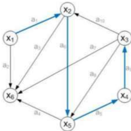
Пути на графе G
