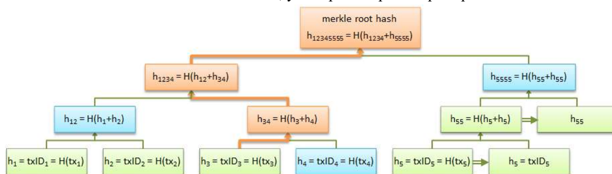
Рис.16.10. Проверка достоверности транзакции с идентификатором txID3
