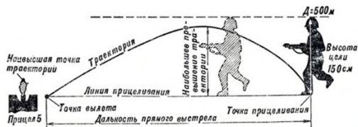
Рис. 3. Прямой выстрел
